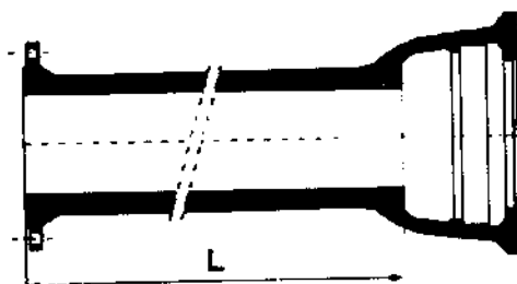
Abrev: TOBF – PN 10 / 16 / 25
